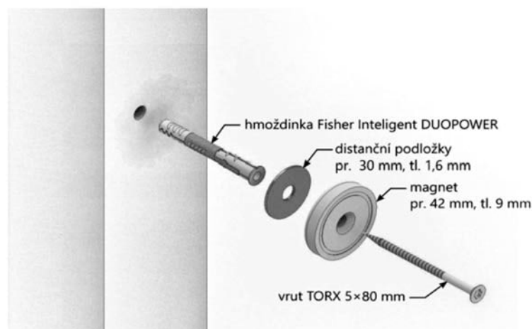
Při využití distančních podložek se použije vrut 90 mm.
