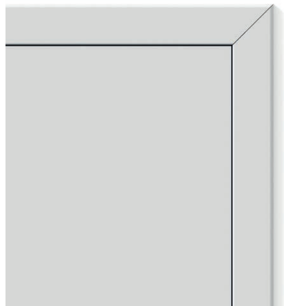
NORMAL Rohový spoj zárubne klasicky pod uhlom 45°.
